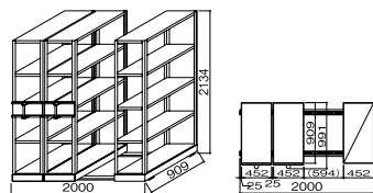
軽量移動ラックプランA 固定1/移動2
