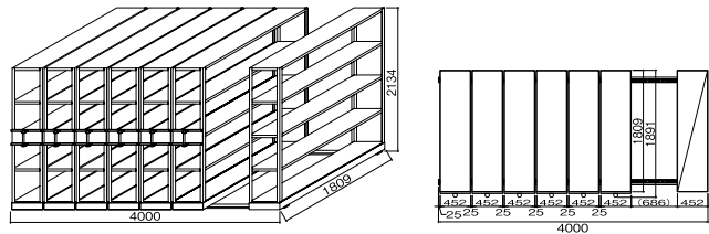
軽量移動ラックプランB 固定1/移動6
