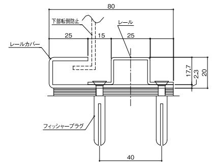
レール断面図
